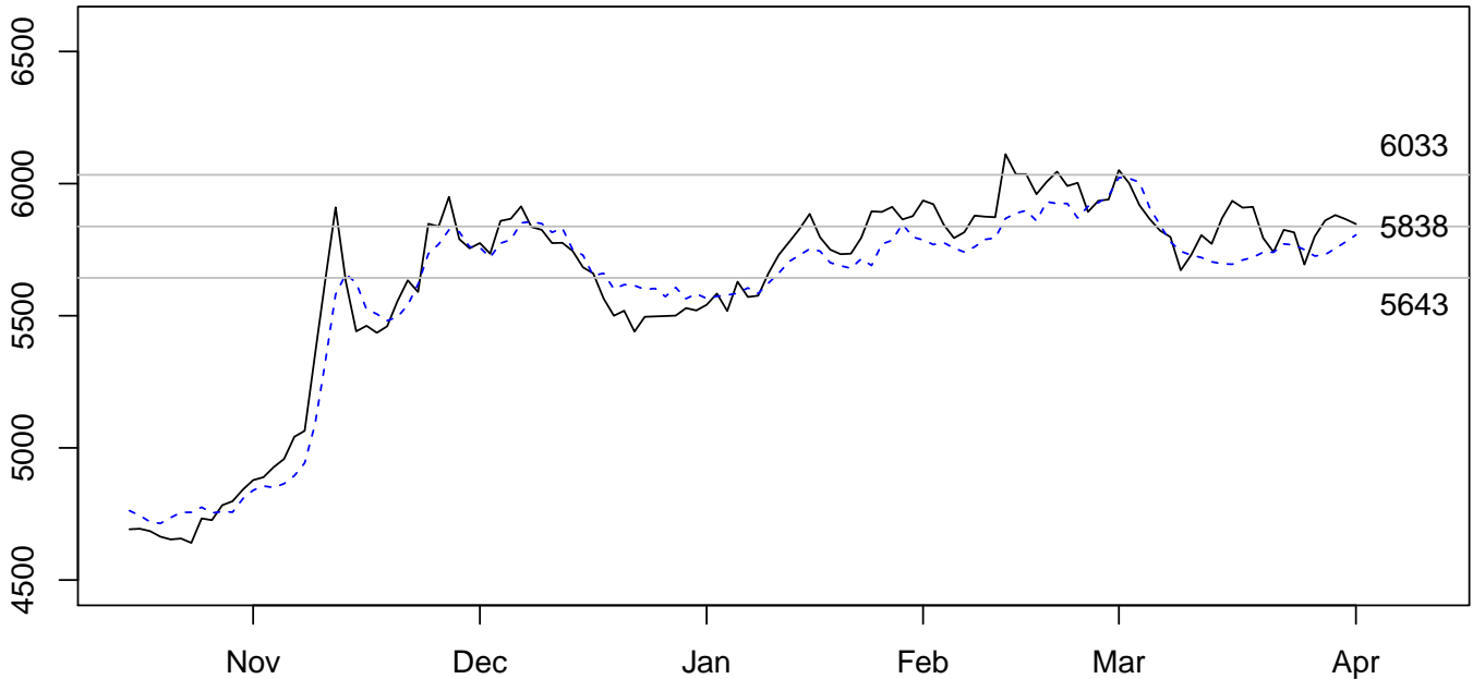
Actual minus Modelled. Last Value = $41 (0.49SD). Last Actual | Modelled Momentum: -1 (orange).
